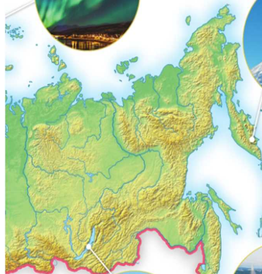
Северное сияние
